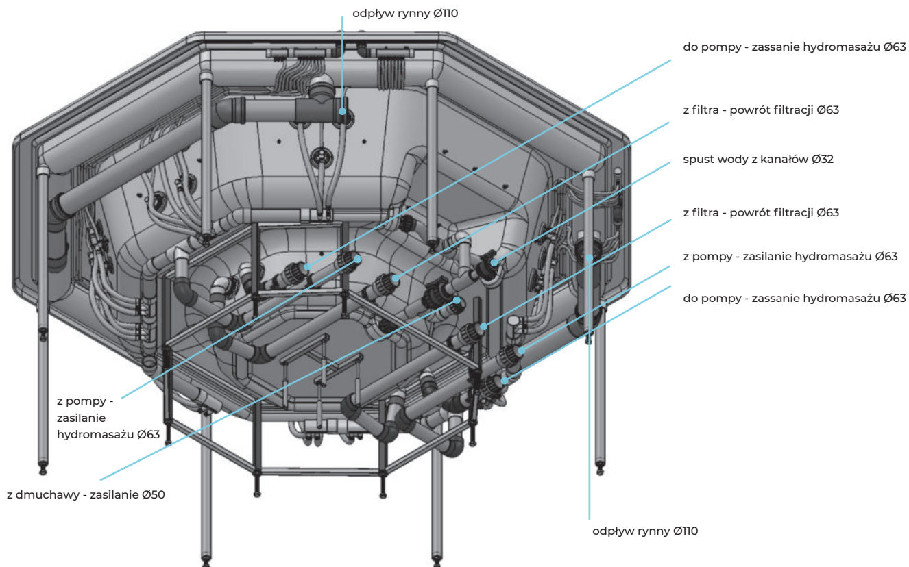
Schemat technologiczny dla wanny SPA z rynną i z 32 dyszami na przykładzie wanny Vesta
