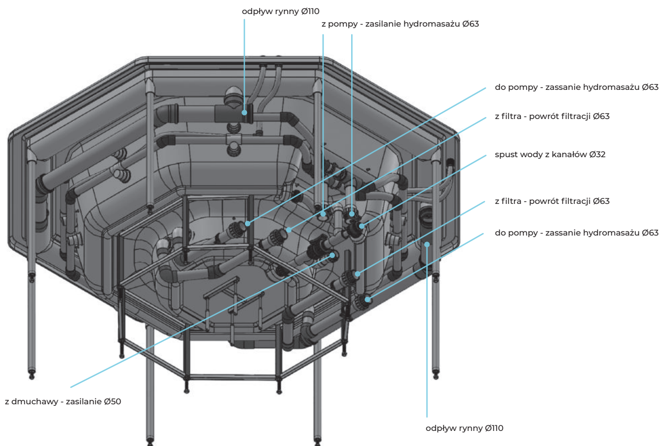
Schemat technologiczny dla wanny SPA z rynną i z podwójnym rzędem dysz na przykładzie wanny Vesta
