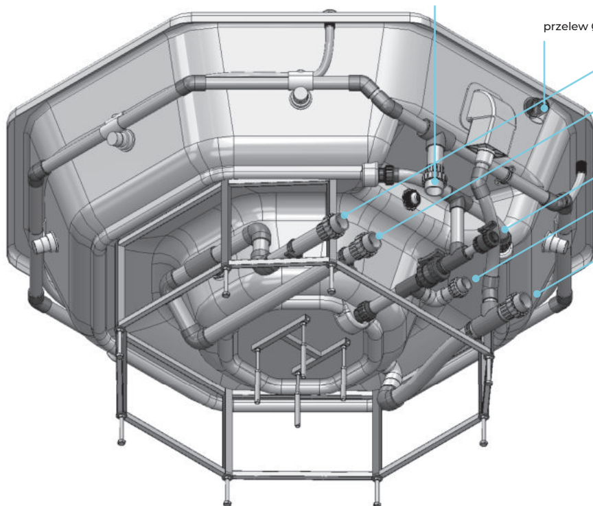
Schemat technologiczny dla wanny SPA ze skimmerem i z pojedynczym rzędem dysz na przykładzie wanny Vesta
