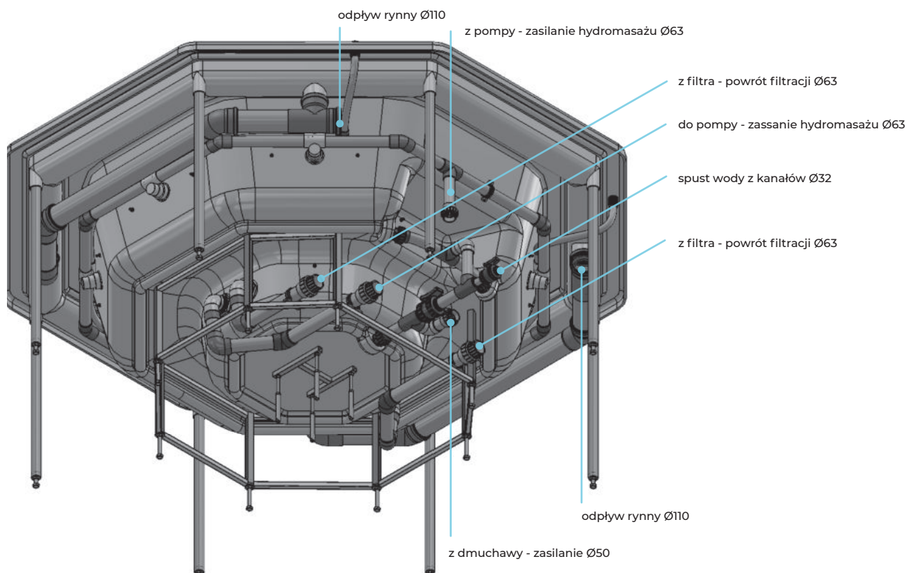
Schemat technologiczny dla wanny SPA z rynną i z pojedynczym rzędem dysz na przykładzie wanny Vesta
